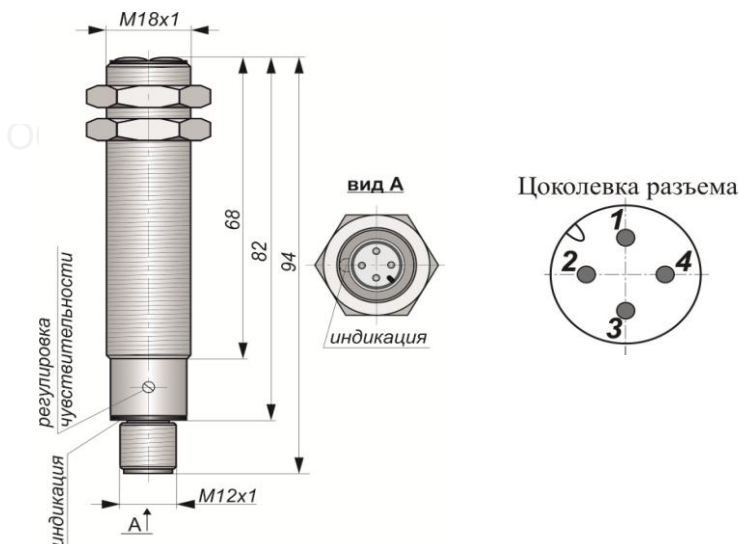
Габаритный чертеж
