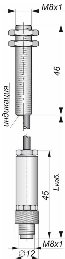
Габаритный чертеж
