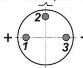
Цоколевка разъема
