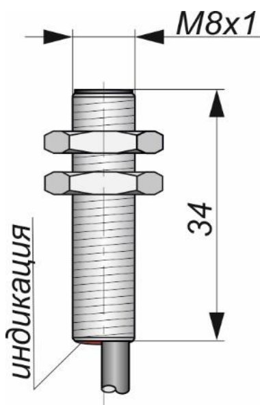
Габаритный чертеж
