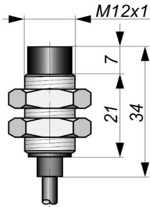
Габаритный чертеж
