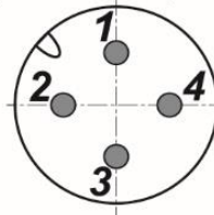
Цоколевка разъема
