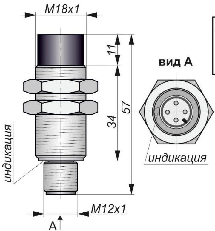
Габаритный чертеж
