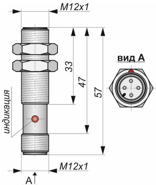
Габаритный чертеж
